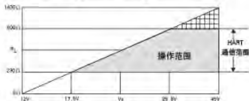
图 3 负载特性图
