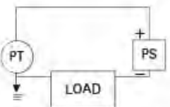
图 3 接地时快速采样计算机在精度上的影响
