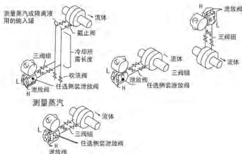
图 16 安装
