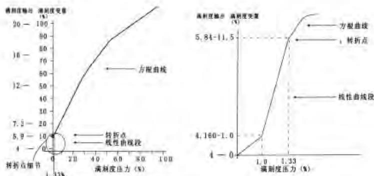
图 2 方根输出曲线
